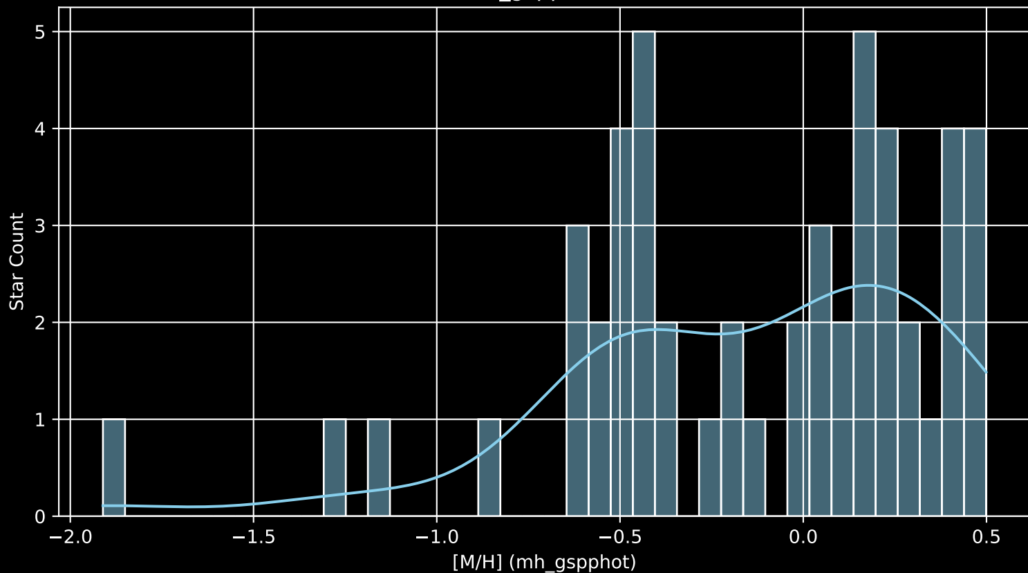
APOGEE DR17 Field: [282-35-O [M/H] (mh_gspphot) (n= 51)
