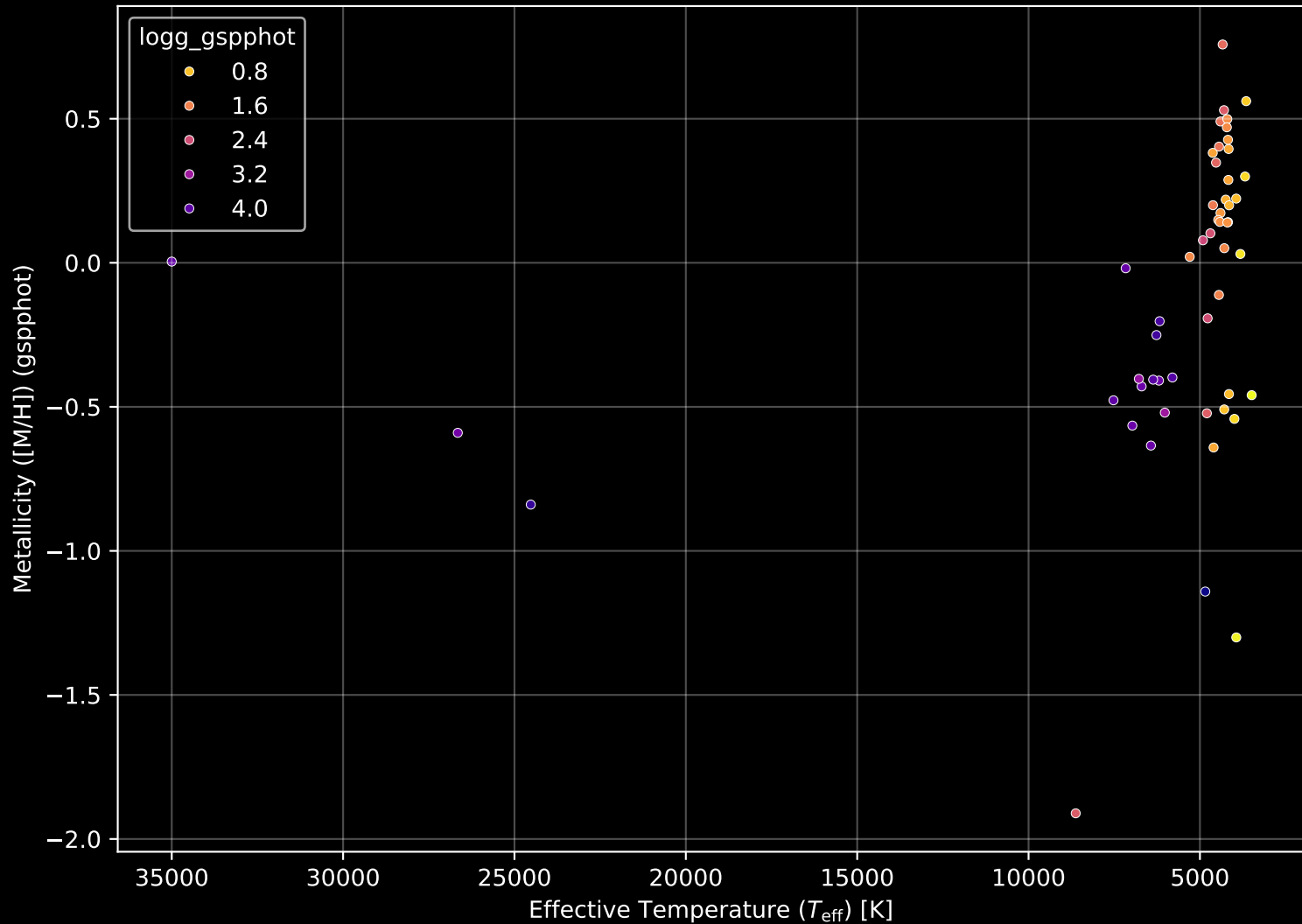
APOGEE DR17 Field: [282-35-O] Stellar Population Parameters (n= 54)
