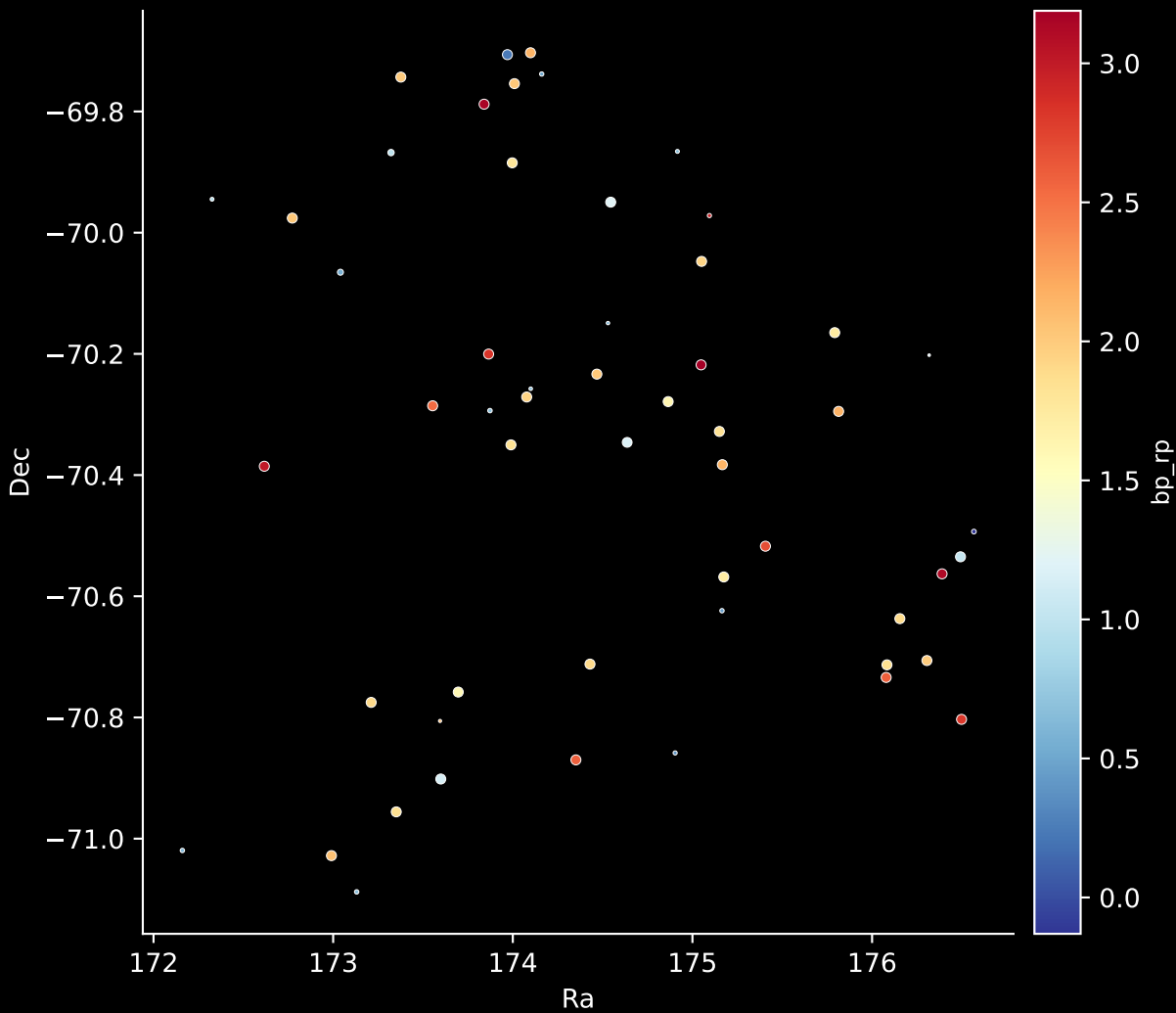
APOGEE DR17 Field: [282-35-O] Stars: 54
